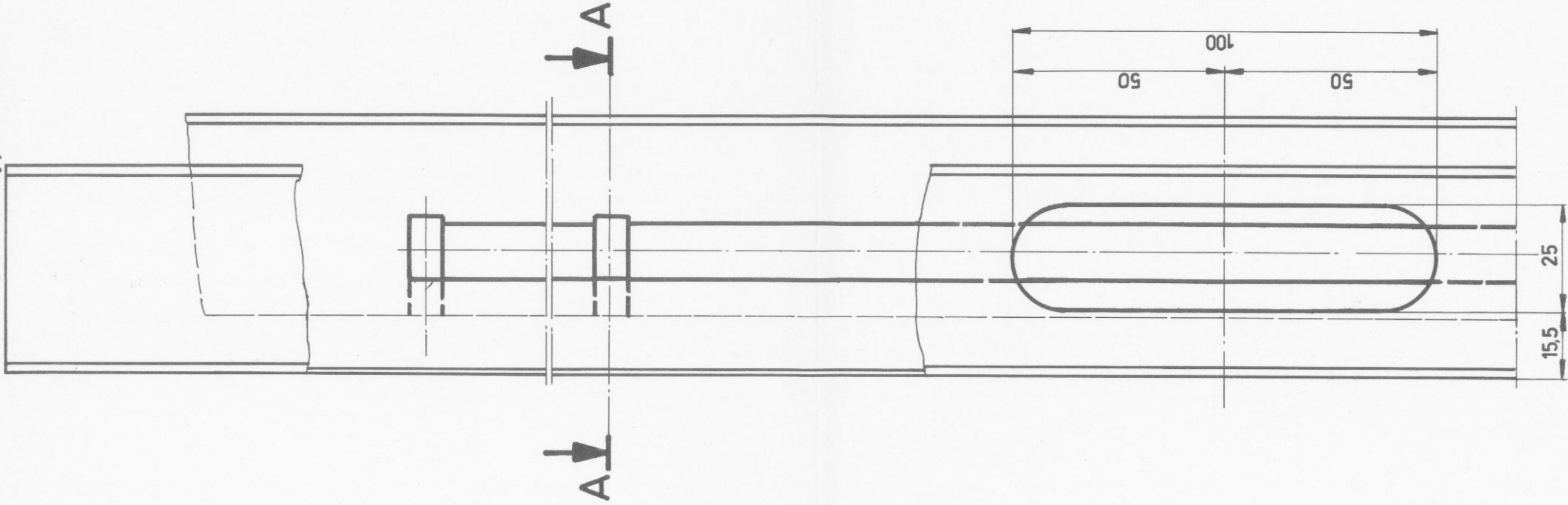
Coupe du haut valable pour types A+B
