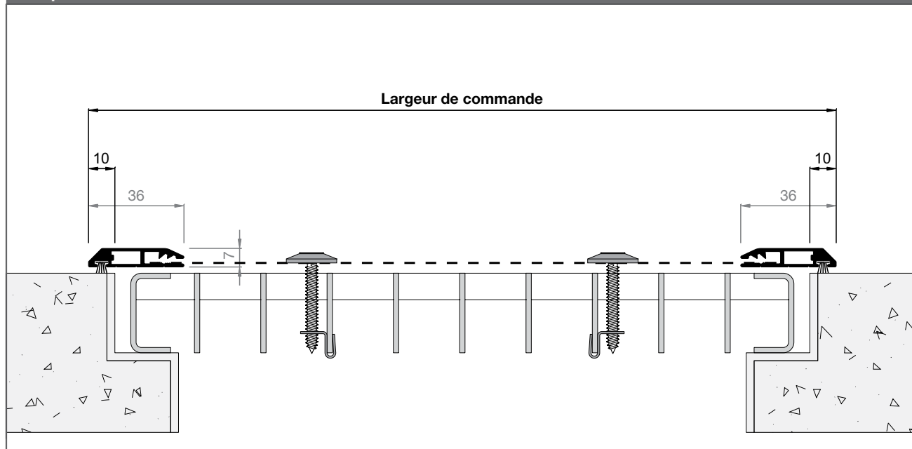
Coupe horizontale
