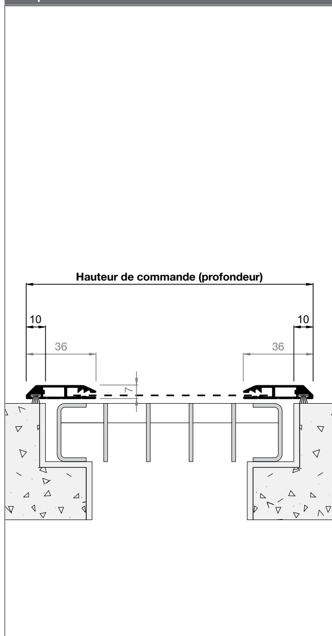
Coupe verticale
