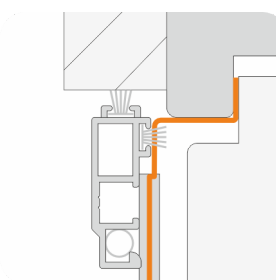
1141SR avec crochet en Z
