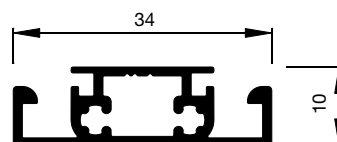
A1.2018 Traverse divisant la toile
