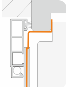
1340SR avec crochet en Z
