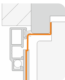
1340SR avec crochet en Z
