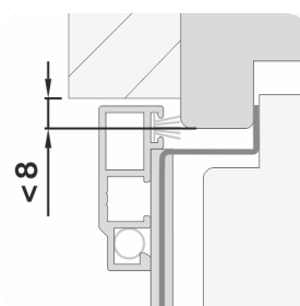
1141SR avec crochet standard
