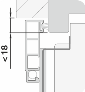
1340SR avec crochet standard
