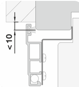
1141SR avec crochet standard
