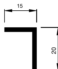
A9.1001 L-Schiene
