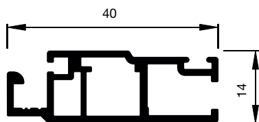
A1.2016 Drehtürprofil
