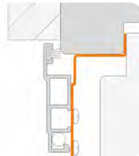
1141SR mit Z-EHW
