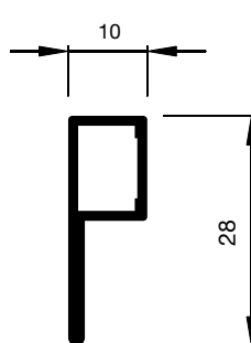
A1.3002 P-Schiene
