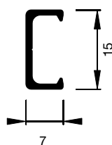
A5.6018 Montageprofil
