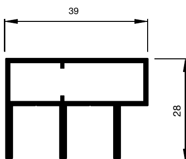
A1.3008 W-Schiene
