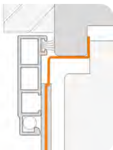
1340SR mit Z-EHW
