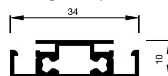
A1.2003 Sprosse gewebeteilend
