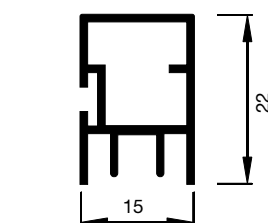
A5.6004 Frontmontageprofil
