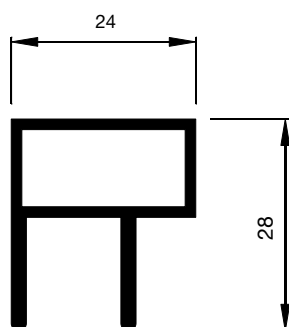
A1.3006 U-Schiene
