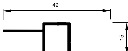
A1.2021 Montagerahmenprofil FV
