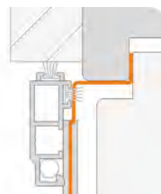
1141SR mit Z-EHW
