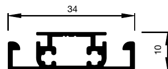
A1.2018 Sprosse gewebeteilend
