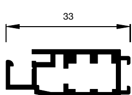
A1.2000 Pendeltürprofil
