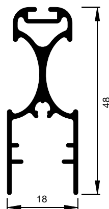
A5.6001 Griffprofil
