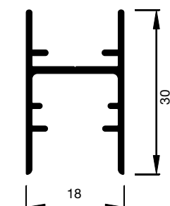
A5.6017 H-Profil
