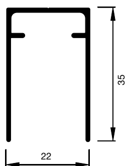
A5.6002 Führung oben
