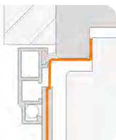
1340SR mit Z-EHW
