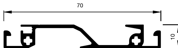
A1.2020 Griffsprossenprofil
