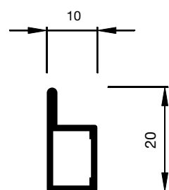
A1.3003 p-Schiene
