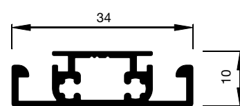
A1.2018 Sprosse gewebeteilend
