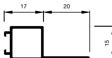
A1.2002 Montagerahmenprofil PT2/PT4
