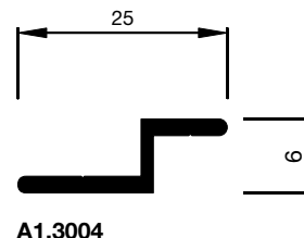
A1.3004 z-Schiene
