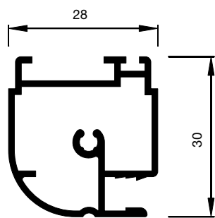
A1.2011 Drehtürprofil
