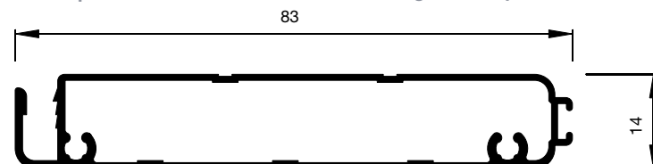
A1.2013 Trittschutzprofil
