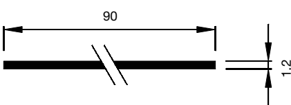
A1.2005 Trittschutzprofil
