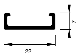
A5.6003 Bodenprofil
