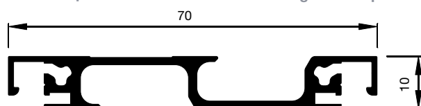
A1.2004 Griffprofil
