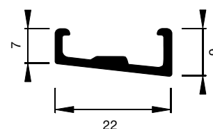
A5.6019 Bodenprofil schräg
