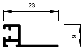
A1.2019 Bürstsenprofil
