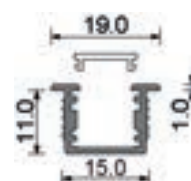
60.188.22 Abbildung mit Endkappe
