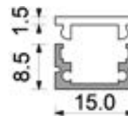
60.188.05 Illustration avec capuchon
