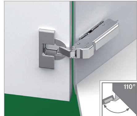
Illustration avec caches protecteurs pour bras de charnière <br/>et boîtier de charnière. A commander séparément.
