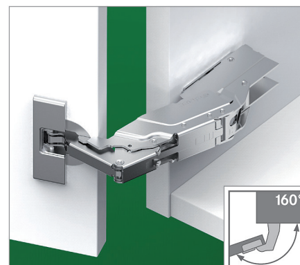
Illustration avec caches protecteurs pour boîtier de charnière. A commander séparément.
