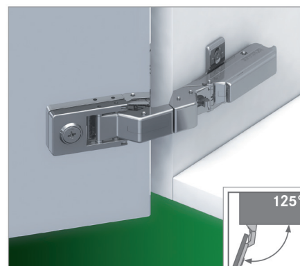
44.076.11-12 sans cache protecteur
