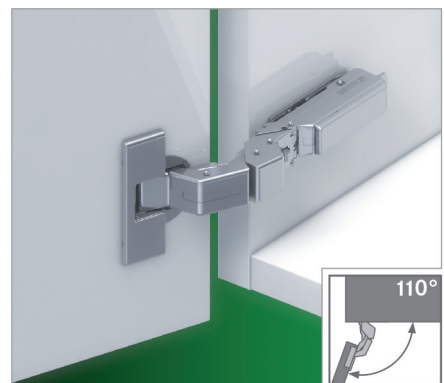
Illustration avec cache protecteur pour bras de charnière. A commander séparément.
