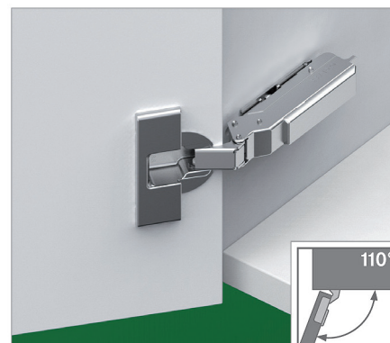
Illustration avec caches protecteurs pour bras de charnière et boîtier de charnière. A commander séparément.
