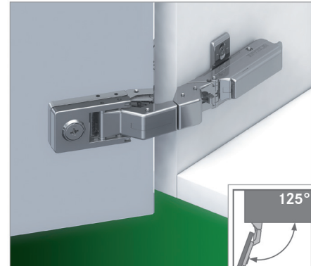
44.076.15 sans cache protecteur
