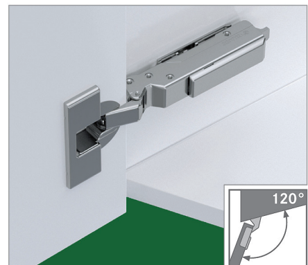
Illustration avec caches protecteurs pour bras<br/>de charnière et boîtier de charnière. A commander séparément.
