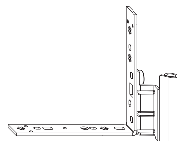
34.408.13-34 ohne ÜV, Abbildung = rechts
