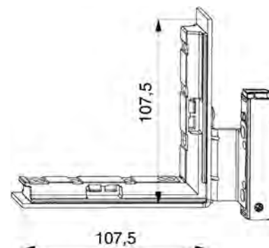
34.408. / 34.418. mit ÜV und WBU Abbildung = rechts
