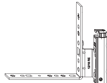
34.408. / 34.418. mit ÜV Abbildung = rechts
