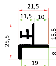
Zargenprofil TFN
