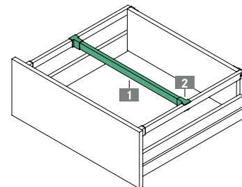
58.270.01-03 mit Halter 58.270.91-93 auf Rechteckreling
