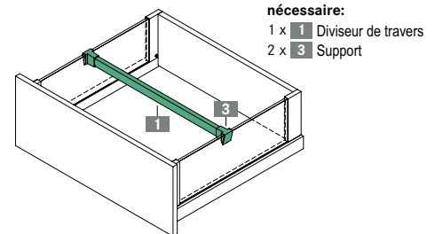
58.270.01-03 avec support 58.270.91-93 sur tube rectangulaire
