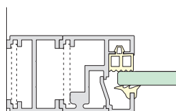
AT 44 - Festverglasung mit Zusatzprofil
