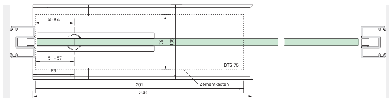
Grundriss / Pendeltür mit BTS 75 V
