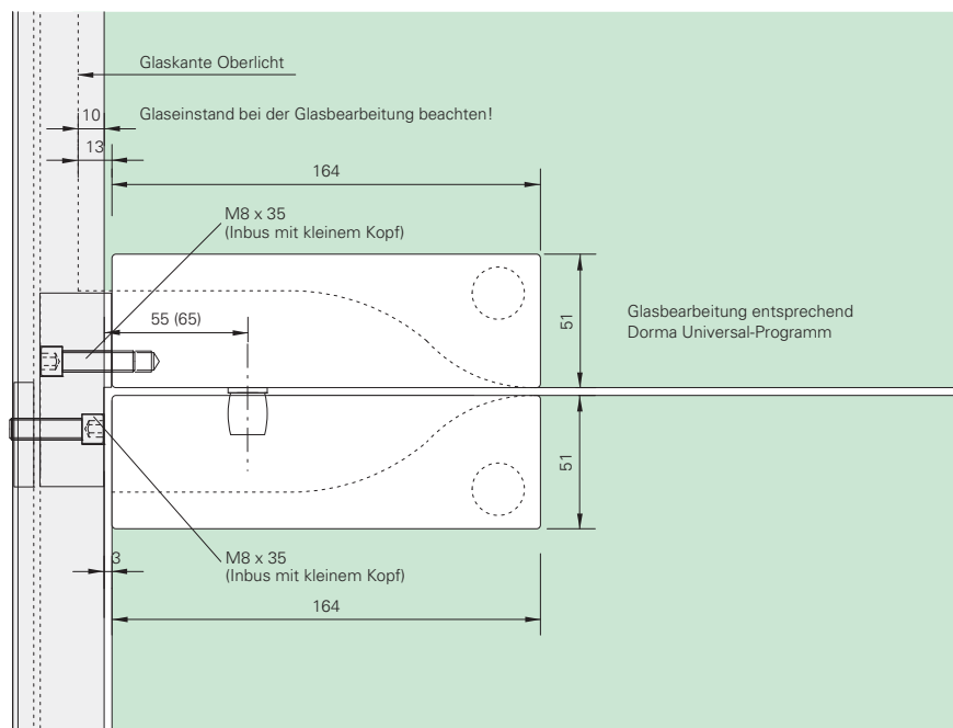
Ansicht Dorma Universal-Band
