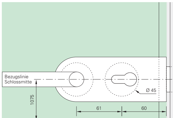
Ansicht Studioschloss, Rondo
