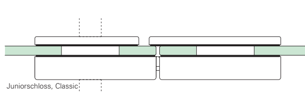
Ansicht Juniorschloss, Classic mit Gegenkasten
