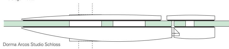
Ansicht Arcos Studioschloss mit Gegenkasten
