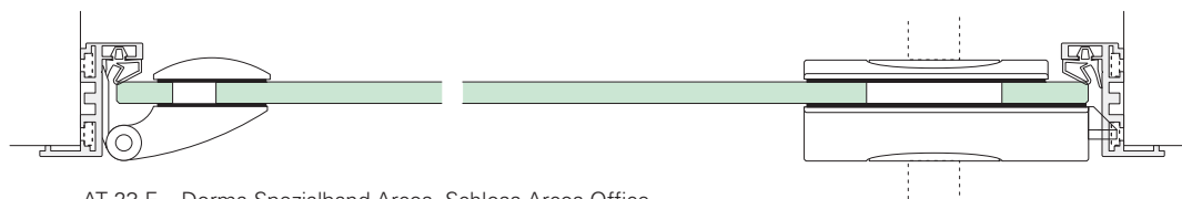
AT 23 E – Dorma Spezialband Arcos, Schloss Arcos Office
