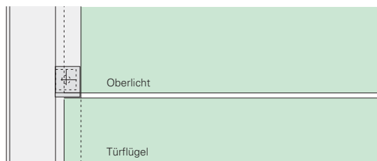
Oberlichtbefestigung Haltenwinkel justierbar
