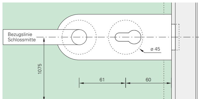
Ansicht Studioschloss
