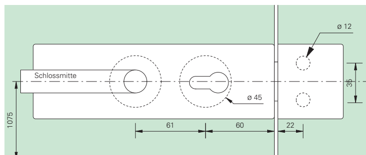
Ansicht Arcos Studioschloss mit Gegenkasten
