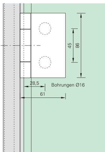
Spezialtürband, Classic / Glasbearbeitung
