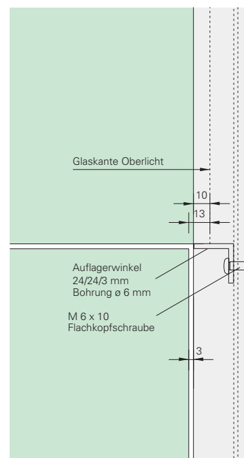
Ansicht Auflager – Oberlicht
