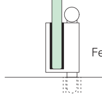
Sprossenprofil für AT44 Zargenrahmen
