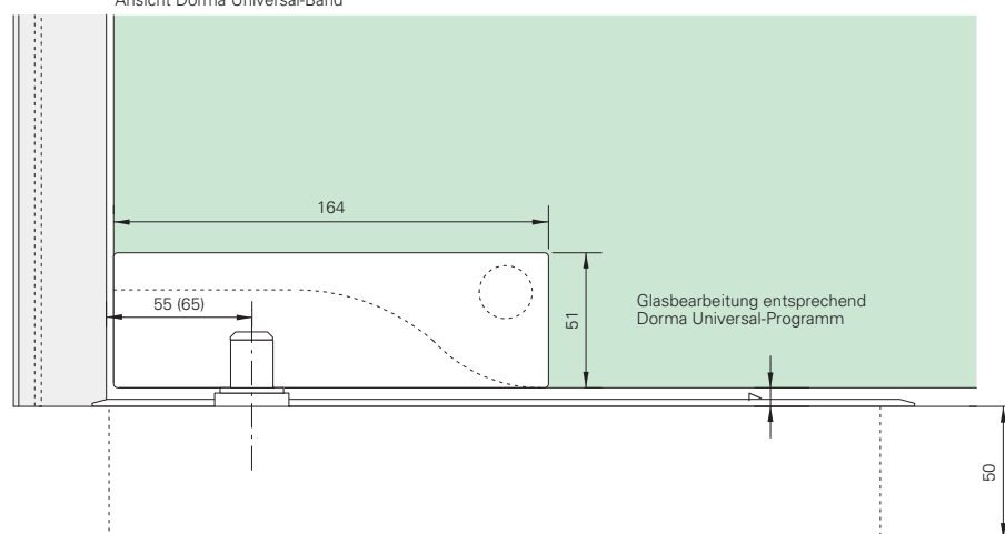
Ansicht Dorma Universal-Band, Bodentürschliesser
