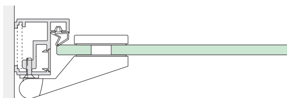
Junior-Variante mit Anschraubband
