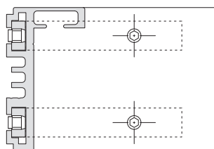
Gehrungsverbindung mit Eckwinkel
