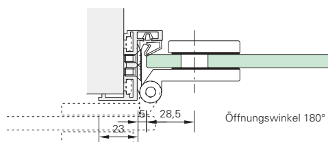
Grundriss
