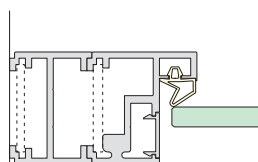
AT 44 - mit Zusatzprofil
