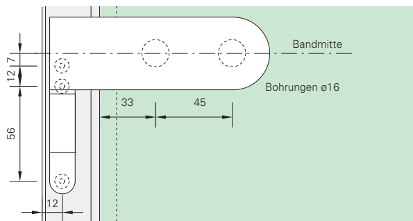
Oberlichtbefestigung Haltenwinkel justierbar
