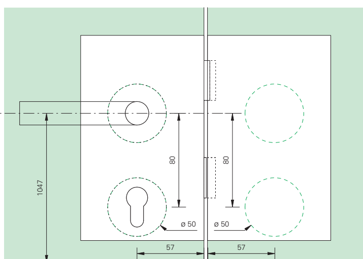
Ansicht Juniorschloss, Classic mit Gegenkasten
