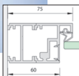
► AT 44EA Anschlagtürzarge
