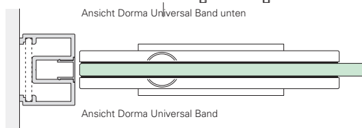
Grundriss
