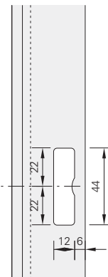
Fräsbild Türfalle
