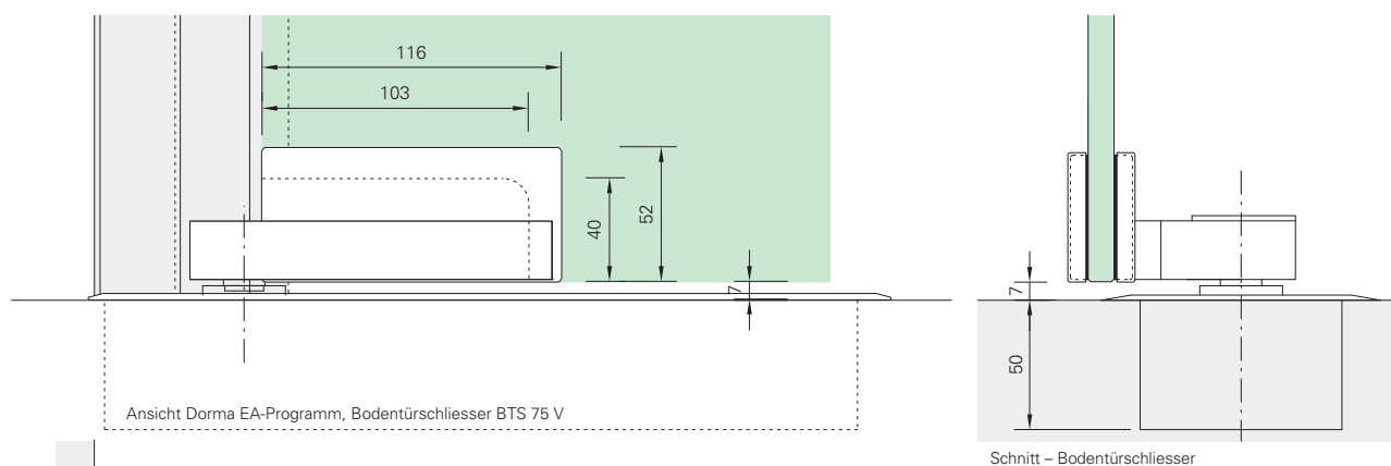
Schnitt – Bodentürschliesser
