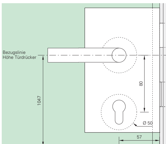
Ansicht Juniorschloss, Office Classic
