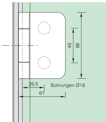
Spezialtürband / Glasbearbeitung
