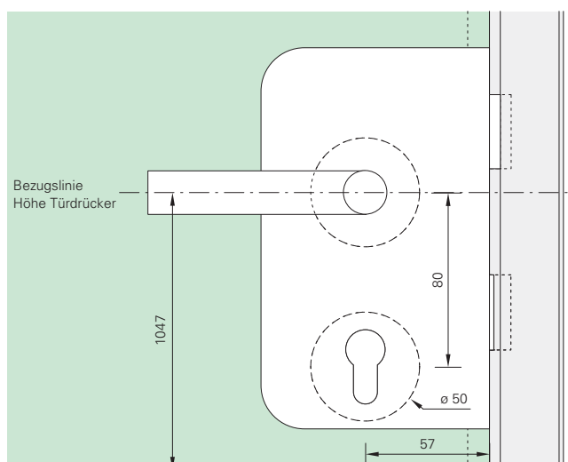
Ansicht Juniorschloss
