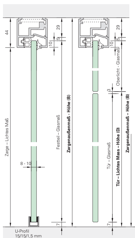
Schnitt
