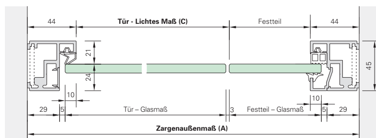
Grundriss / Tür mit Festverglasung
