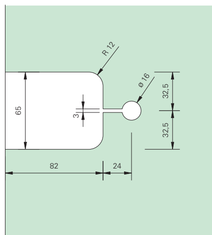
Glasbearbeitung Dorma - Tensor Programm
