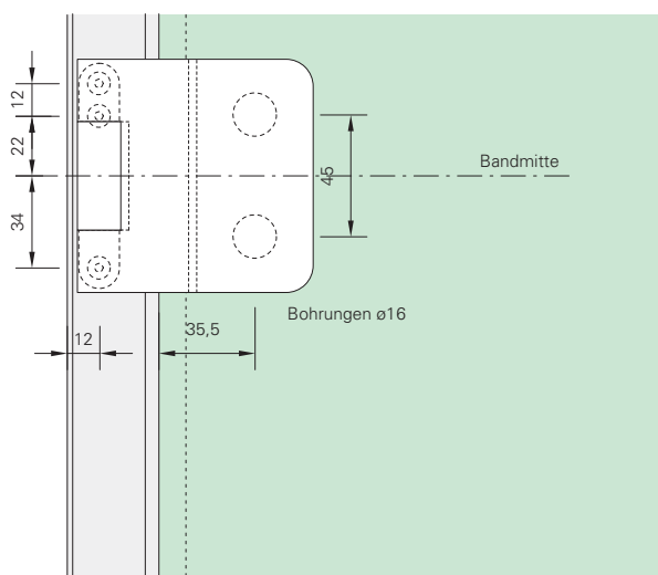
Studio-Variante mit Anschraubband
