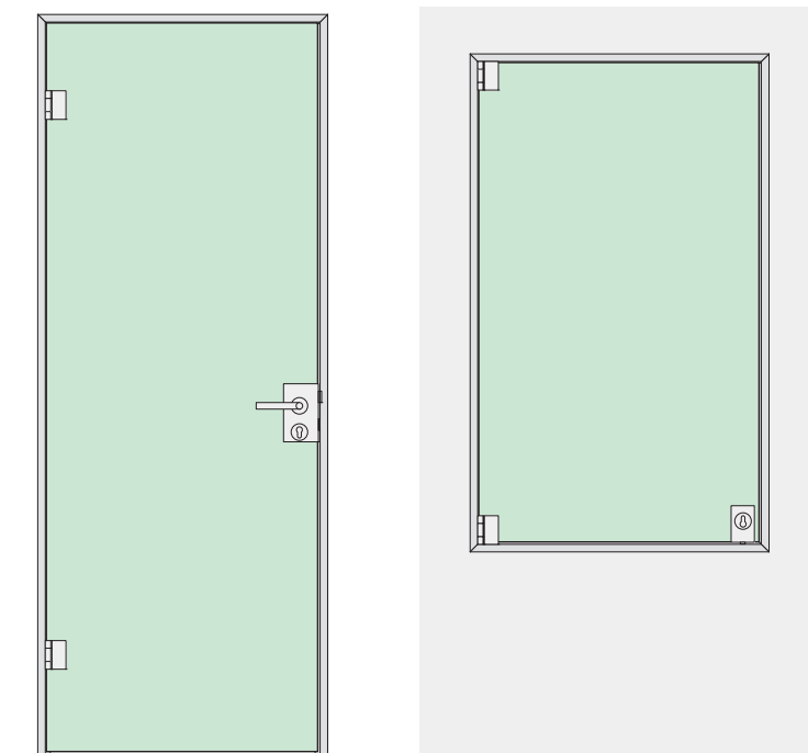
AT 23 E – Eckanschlagtürzarge
