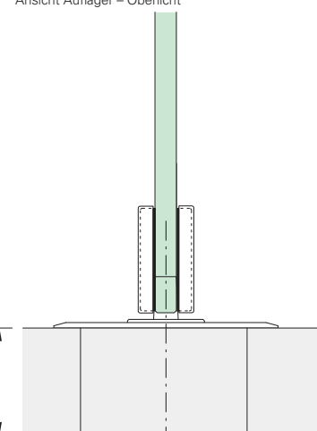
Schnitt – Bodentürschliesser
