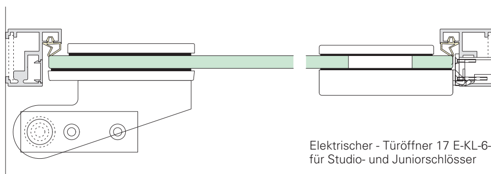
AT-44, Dorma EA-Program - Bodendrehlager
