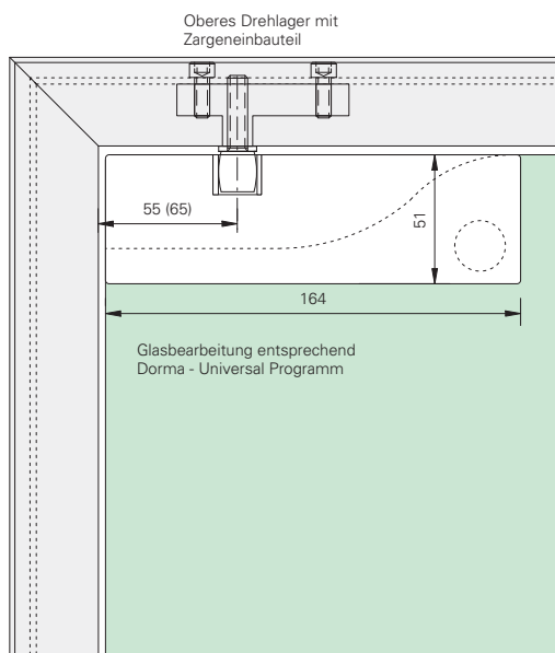
Ansicht Dorma Universal Band oben
