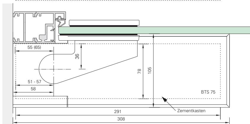
Schnitt – Bodentürschliesser
