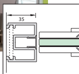
► PT 35 Pendeltürzarge
