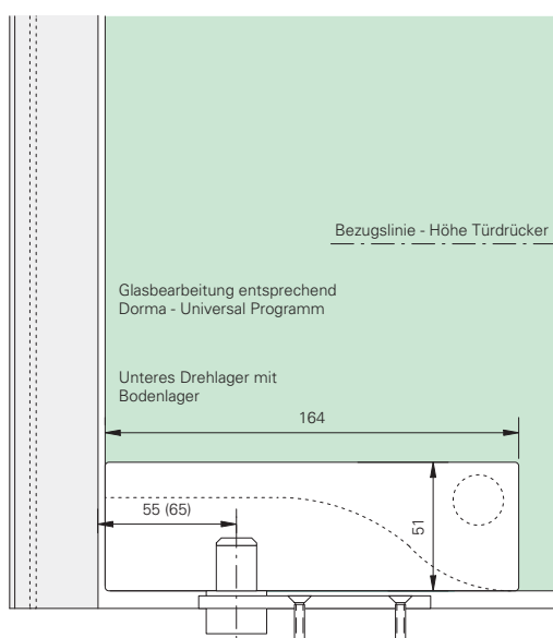
Ansicht Dorma Universal Band unten
