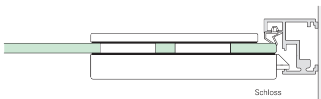
Ansicht Studioschloss
