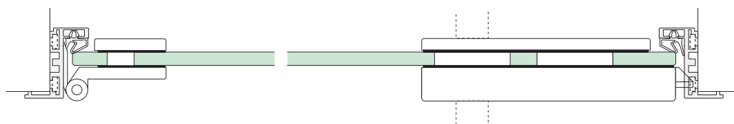
AT 23 E – Dorma Spezialband, Studioschloss (Rondo, Classic)
