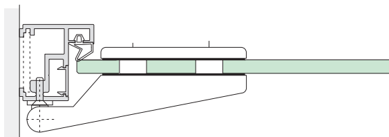
Studio-Variante mit Anschraubband
