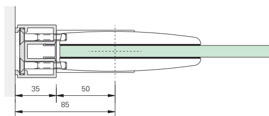
Grundriss
