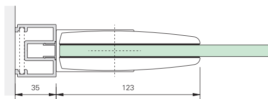
Grundriss
