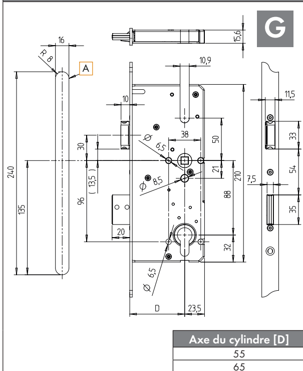
Coffre principal type G, axe cylindre 55 et 65, entraxe 88
