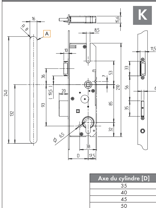
Coffre principal type K, axe cylindre 35-50, entraxe 85 mm
