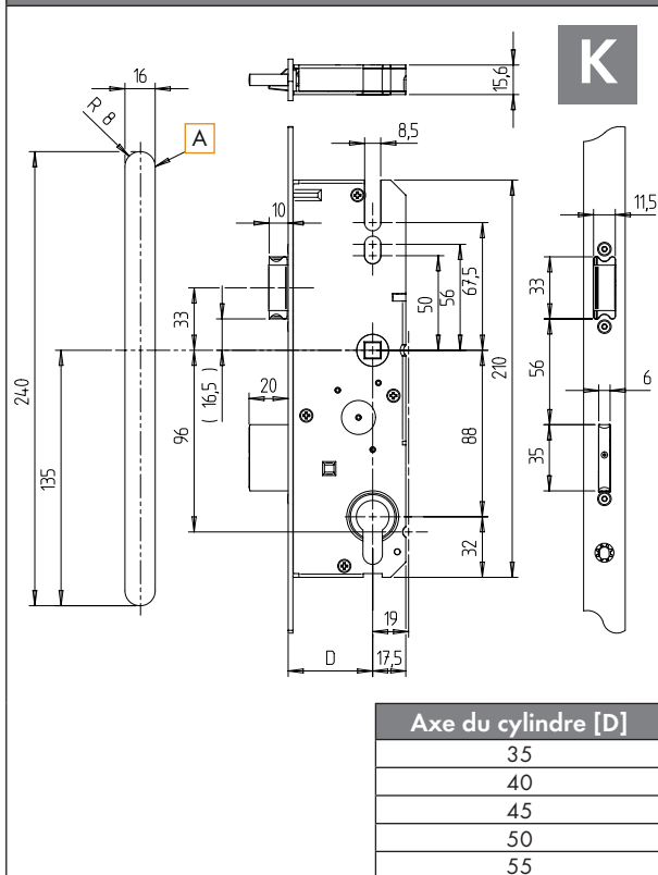
Coffre principal type K, axe cylindre 35-55, entraxe 88 mm
