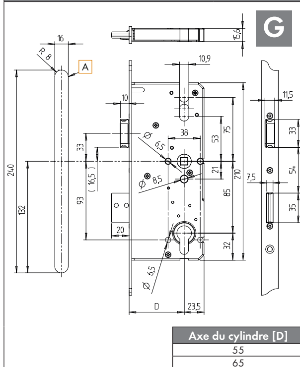
Coffre principal type F, axe cylindre 55 et 65, entraxe 85
