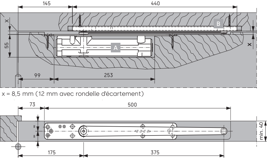
Exemple d'installation ITS Home avec glissière G 96 N20 dans une porte à panneau plein
