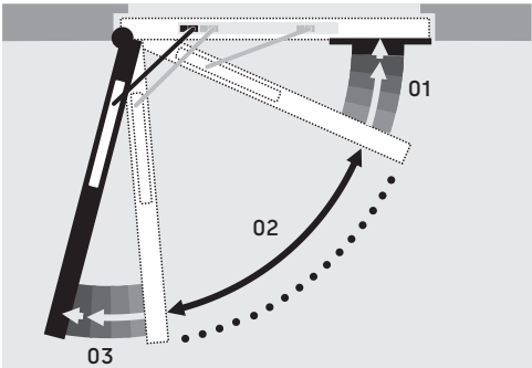
Exemple d'installation ITS Home avec glissière G 96 N20 dans une porte à panneau plein
